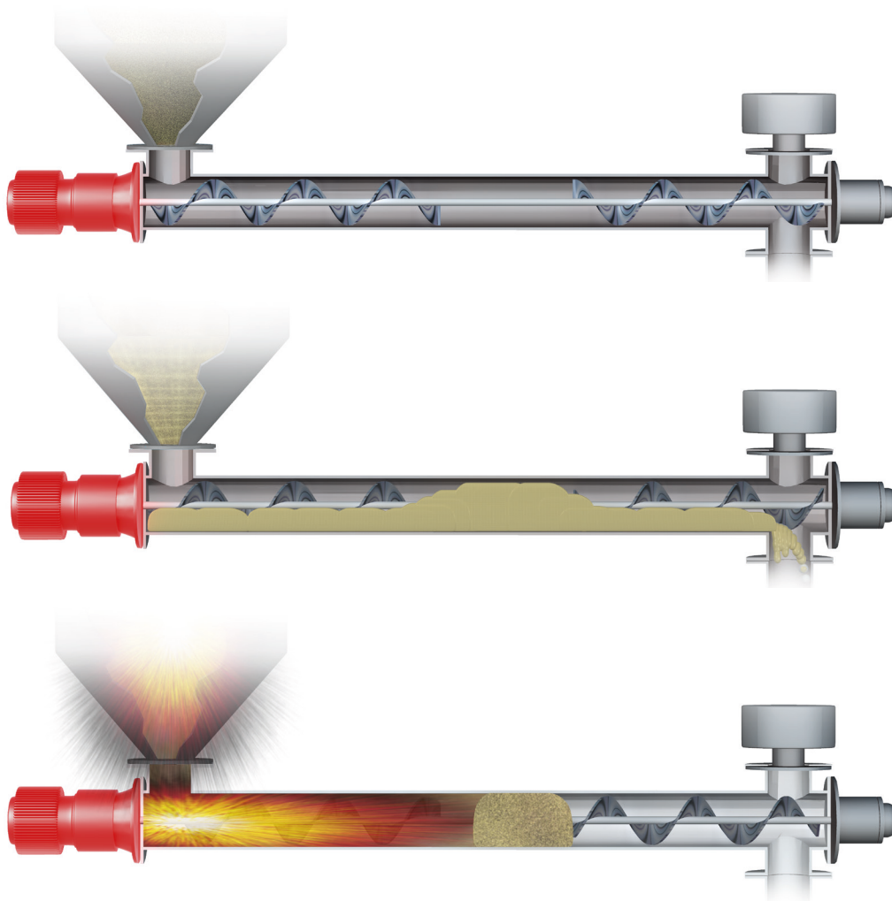
Bild 16: Verwendung einer Rohrförderschnecke zur explosionstechnischen Entkopplung Erzeugung eines Schüttgutpfropfens durch Entfernung von 1, 1\frac{1}{2} oder 2 Wellengängen. Der Pfropfen soll möglichst auch dann bestehen bleiben, wenn beim Leerfahren kein Schüttgut mehr zugeführt wird.
