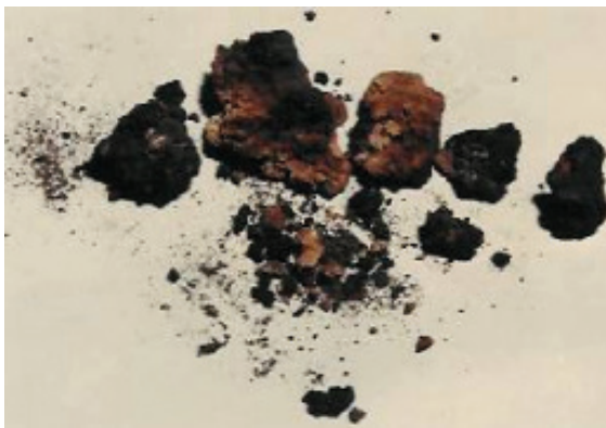
Bild 9: Verkohltes Produkt aus dem Motorraum eines Radladers (Bild: Prof. Siegfried Radandt)
