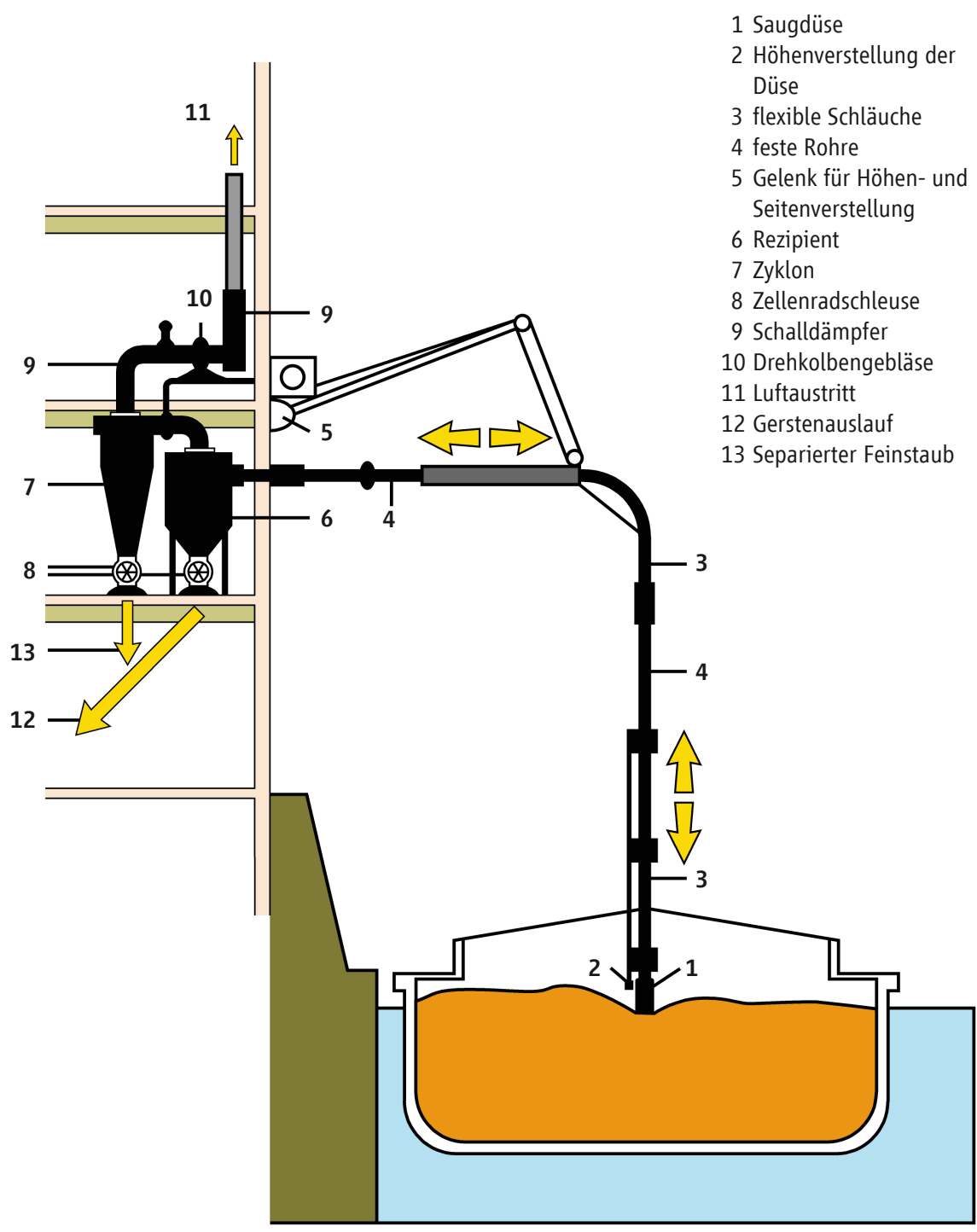
Bild 6: Schematische Darstellung einer Schiffsentladung (Gerstenannahme)
