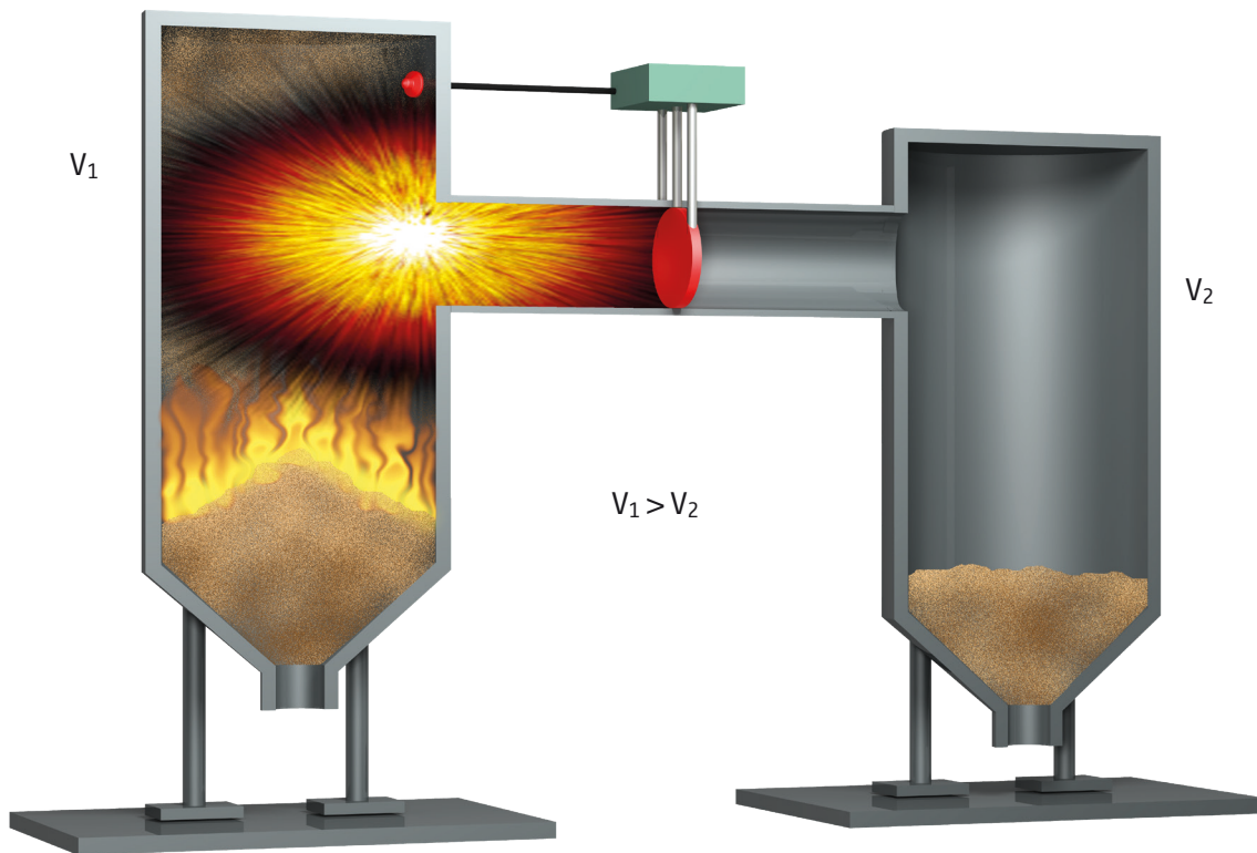
Bild 13: Verhindern einer Explosionsübertragung über eine Rohrleitung durch eine notwendige Entkopplung mittels Schnellschlusschieber
